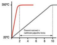
Průběh nahřívání taveniny
